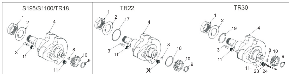
21 - CONJUNTO VIRABREQUIM
